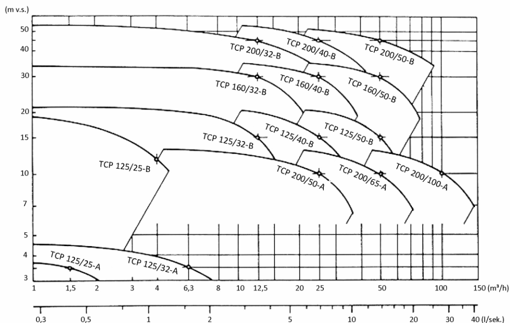
Karakteristika Q-H:
